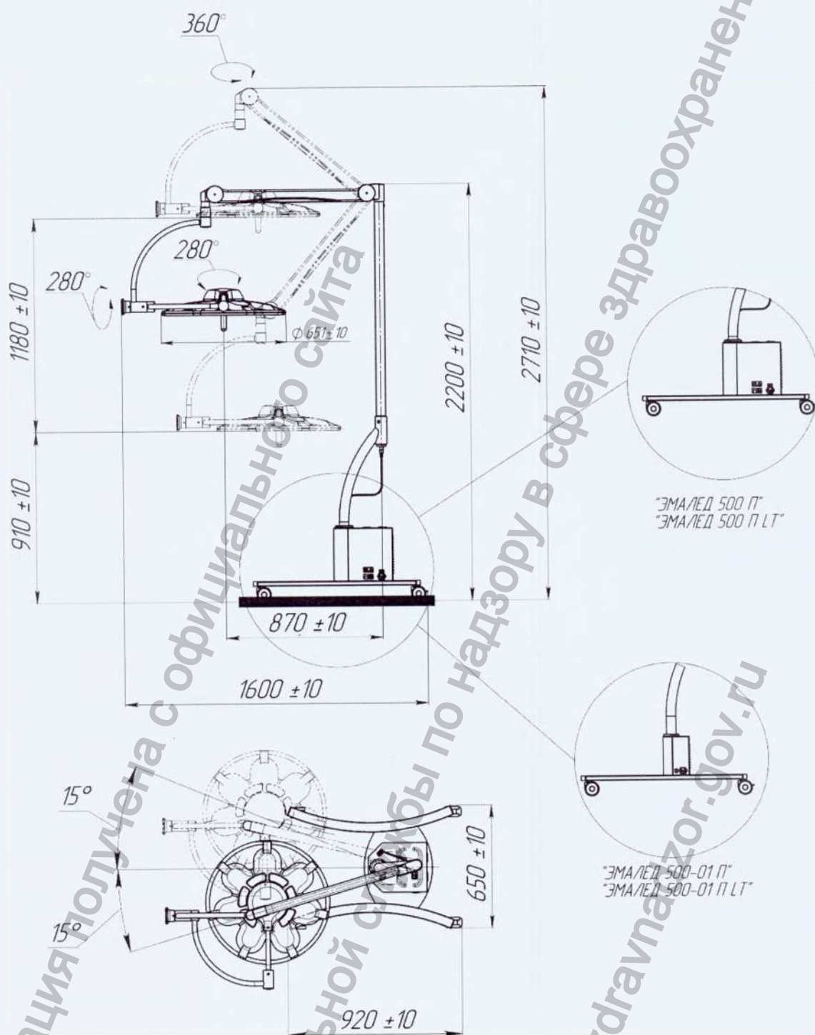
Рисунок А.32 – Габаритные размеры и параметры перемещения
