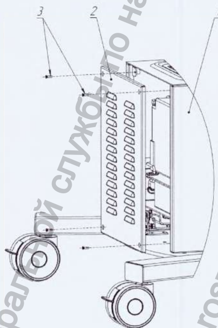
Рисунок А.3 – Установка блока питания на опору
