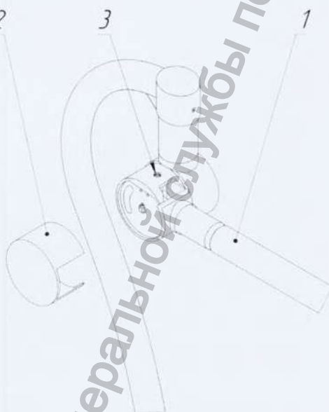
Рисунок А.12 – Монтаж блоков освещения с одним дуговым шарниром
