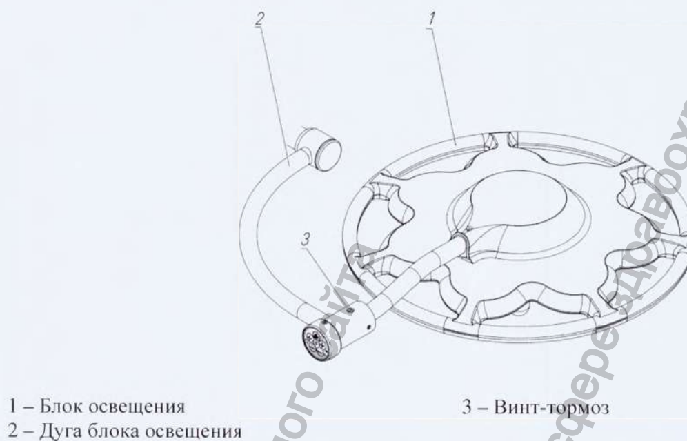
Рисунок А.13 – Настройка усилия поворота блока освещения
