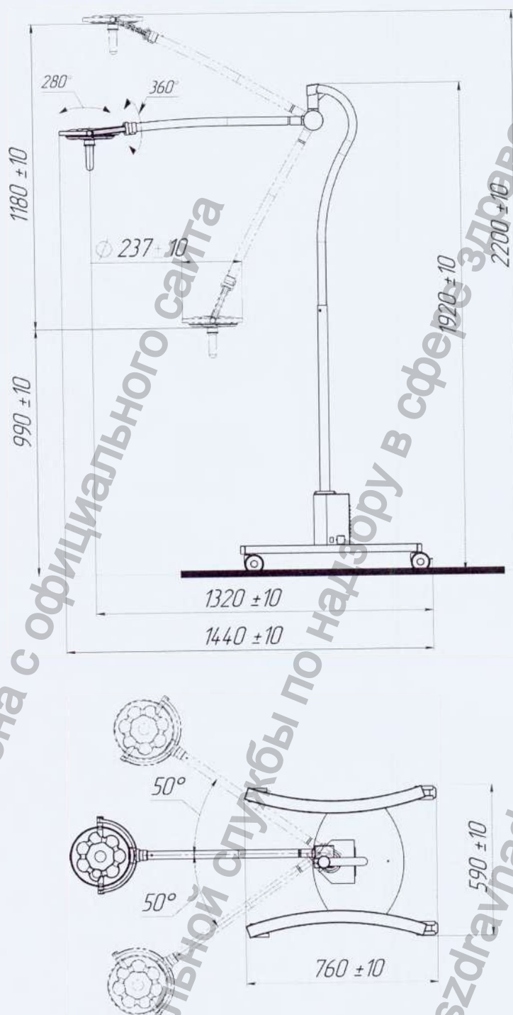
Рисунок А.23 - Габаритные размеры светильника «ЭМАЛЕД 200 - 01 П», «ЭМАЛЕД 200 - 01 П LT»
